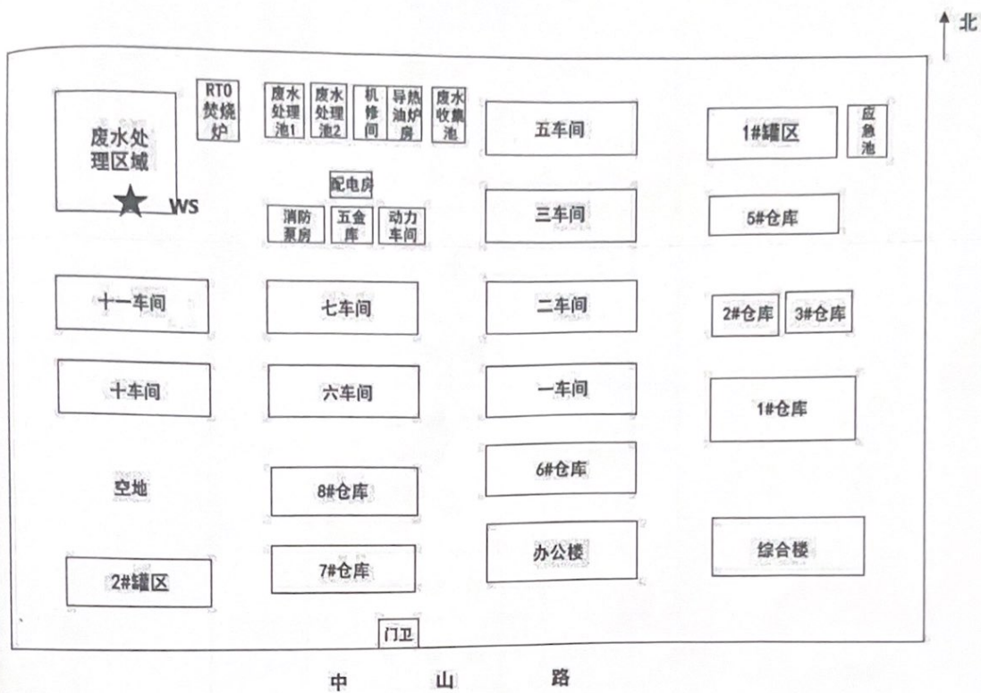
盐城辉煌化工有限公司厂区平面图
