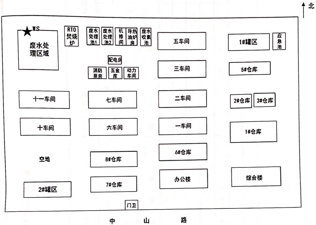
盐城辉煌化工有限公司厂区平面图
